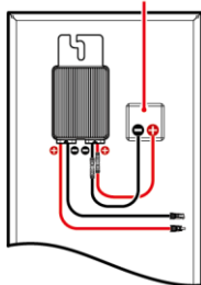
Aansluitkast van de PV-module
